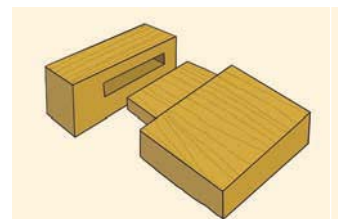
ମର୍ଟିଜା ଓ ଟେନନ୍ ସଂଯୋଗ ସ୍ଥଳ (Mortise and Tenon Joint)
