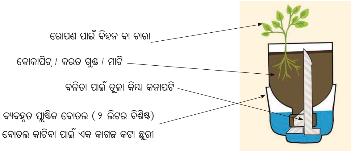
ଚିତ୍ର ୧.୩ (ଖ) ଅବଶୋଷଣ ପ୍ରଣାଳୀ ଆଧାରିତ ହାଇଡ୍ରୋପୋନିକ୍ସ ବ୍ୟବସ୍ଥା
